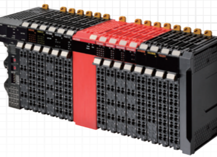
Ведомые терминалы EtherCAT серии NX NX-IO
