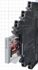
Новинка Тонкие реле ввода/вывода G2RV-SR/G3RV-SR
